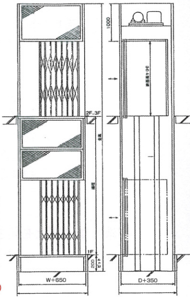
同一方向型 (MC・R) 直行型 (MC・RX)
